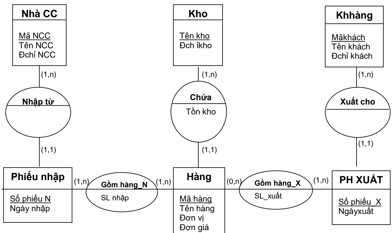
Mô hình thực thể -mối quan hệ của bài toán "QL Kho hàng"
